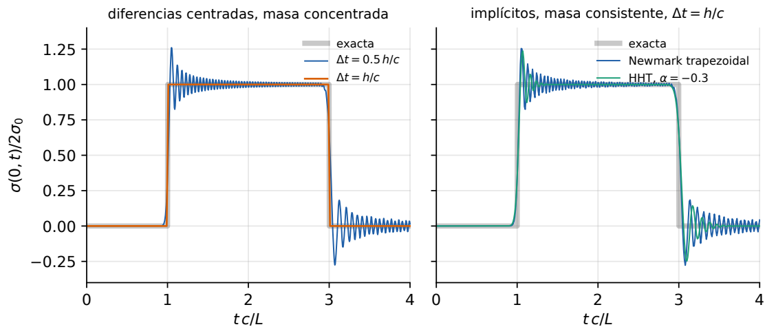
Figura 8.1: Esfuerzo en el empotramiento durante una vuelta de la onda. Izquierda: diferencias centradas con el paso límite y con la mitad. Derecha: Newmark y HHT- \alpha con el paso límite.
