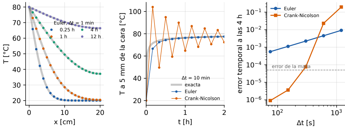
Figura 9.1: Izquierda: perfiles de temperatura a 0.25, 1, 4 y 12 h con Euler implícito y \Delta t = 1 min, sobre la solución exacta (gris). Centro: temperatura a 5 mm de la cara con \Delta t = 10 min. Derecha: error temporal a las 4 h frente al paso, y error de la malla.
