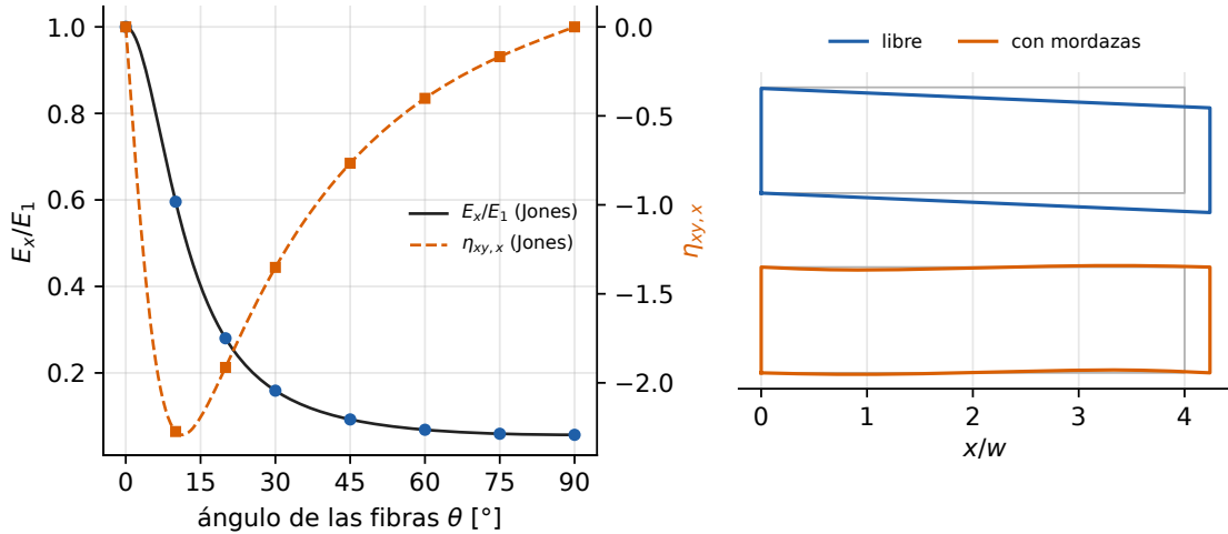
Figura 10.1: Izquierda: módulo aparente y coeficiente de influencia mutua frente al ángulo de las fibras; curvas de la teoría de láminas y puntos de Solidum. Derecha: tira de longitud 4w con las fibras a 45^\circ , libre y con mordazas; las dos deformadas amplificadas hasta el mismo alargamiento.
