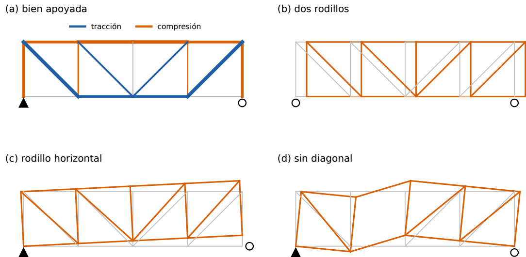
Figura 11.1: (a) Armadura bien apoyada: el grosor de cada barra crece con su fuerza axial; en gris, las barras sin fuerza. (b) a (d): los mecanismos de los tres modelos mal apoyados o mal conectados, calculados con la estática (el núcleo de la matriz de compatibilidad); en gris la geometría inicial y en color el mecanismo, amplificado.
