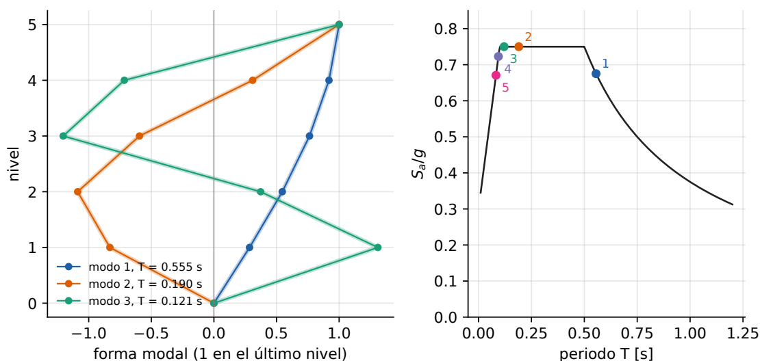
Figura 7.1: Izquierda: los tres primeros modos, Solidum (puntos) sobre los analíticos (bandas). Derecha: el espectro de diseño con los periodos de los cinco modos.
