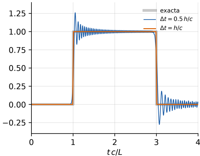
diferencias centradas, masa concentrada
