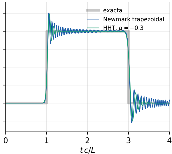
implícitos, masa consistente, \Delta t = h/c
