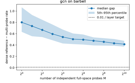
GCN barbell
