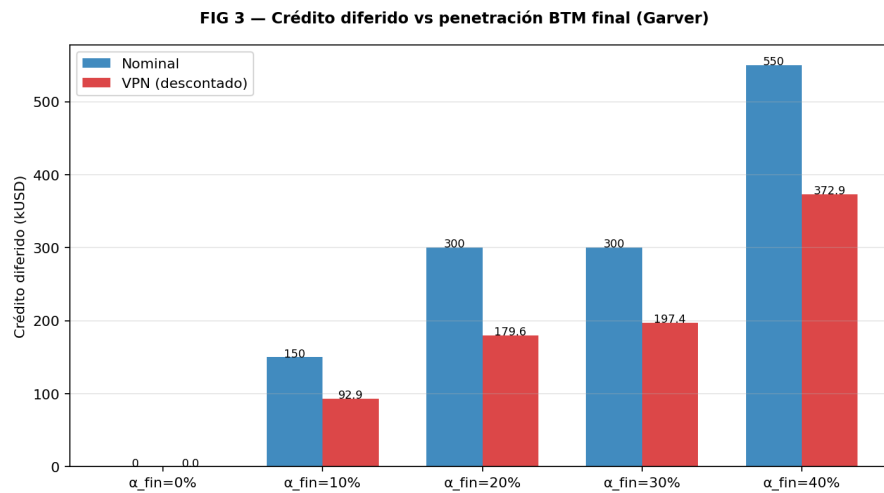
Figura N° 5.14: Crédito diferido nominal y VPN vs. penetración BTM terminal en el sistema Garver. La diferencia entre las barras nominal y VPN representa el efecto del factor de descuento sobre las inversiones postergadas.
