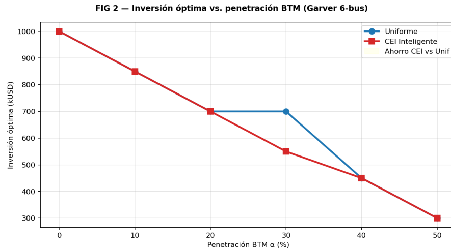
Figura N° 5.3: Inversión óptima vs. penetración BTM en el sistema Garver para las estrategias uniforme y CEI inteligente.
