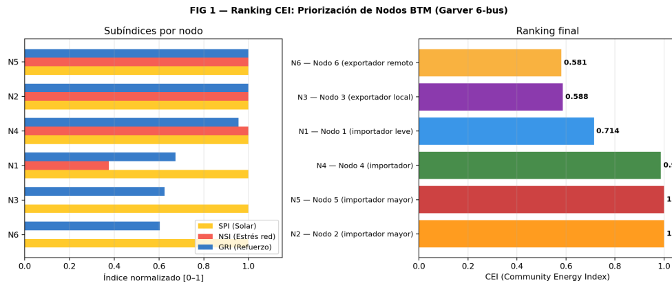
Figura N° 5.2: Ranking CEI de los seis nodos del sistema Garver. Izquierda: descomposición en los subíndices SPI, NSI y GRI. Derecha: índice compuesto CEI ordenado de menor a mayor.
