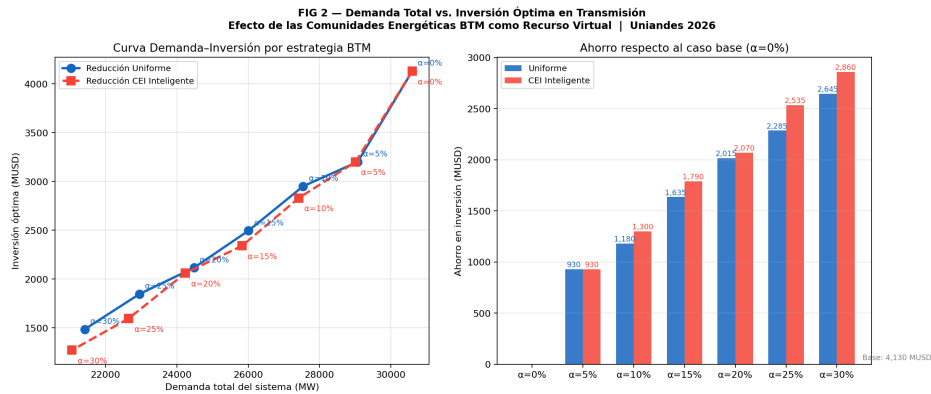
Figura N° 5.8: Inversión óptima vs. penetración BTM en el SIN para las estrategias uniforme y CEI inteligente. También se presenta el ahorro respecto al caso base para diferentes niveles de penetración BTM.
