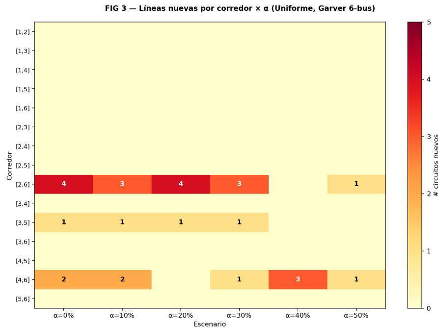
Figura N° 5.4: Matriz de líneas nuevas por corredor y nivel de penetración BTM en el sistema Garver (estrategia uniforme). El color indica el número de circuitos construidos en cada corredor.
