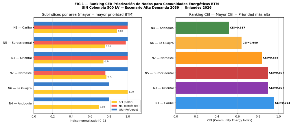
Figura N° 5.6: Ranking CEI de los seis nodos del SIN bajo escenario de estrés. Izquierda: descomposición en SPI, NSI y GRI. Derecha: índice compuesto CEI con identificación de las áreas prioritarias para despliegue BTM.
