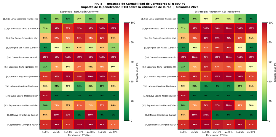
Figura N° 5.10: Mapa de calor de cargabilidad de corredores del SIN para cada nivel de penetración BTM bajo estrategia uniforme.
