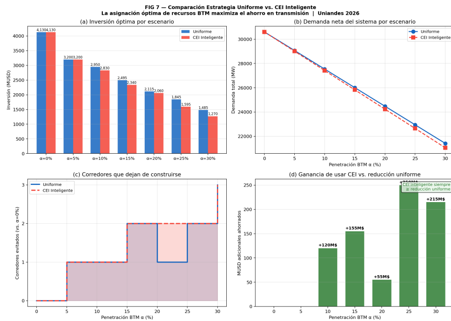
Figura N° 5.11: Comparación de ahorros bajo las estrategias uniforme y CEI inteligente en el SIN para cada nivel de penetración BTM.
