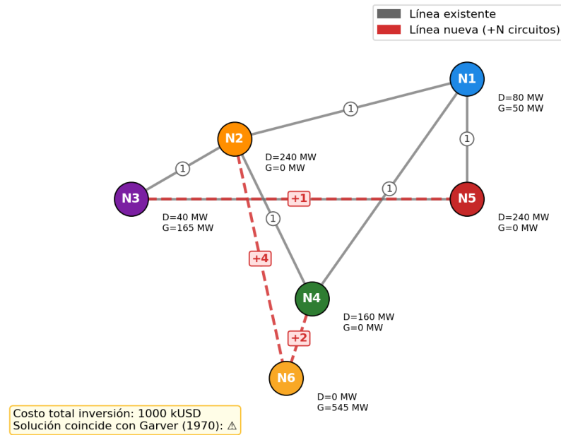
FIG 5 — Topología Garver 6-bus, solución óptima caso base ( \alpha=0\% )
