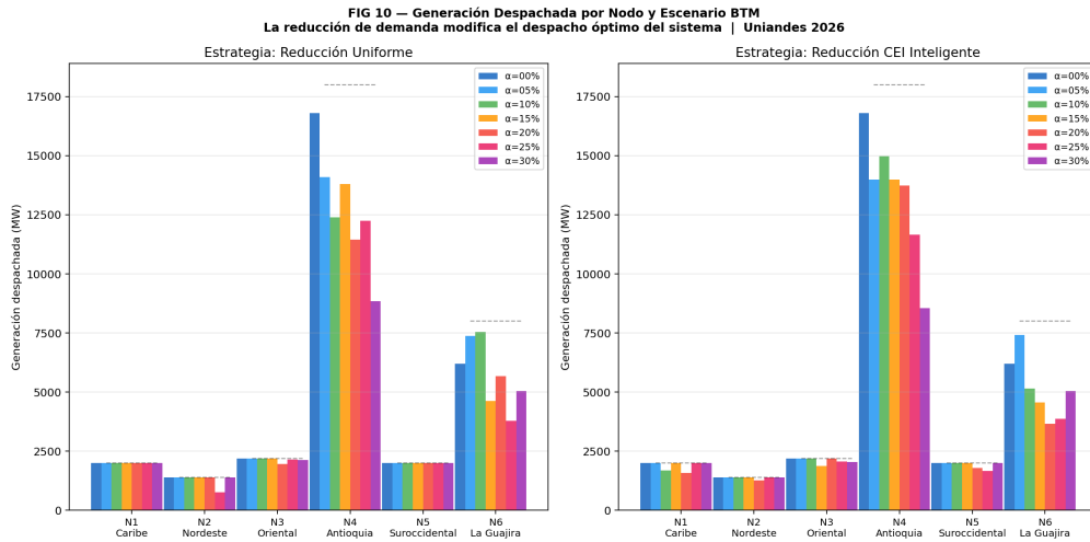
Figura N° 5.12: Generación despachada por nodo y nivel de penetración BTM en el SIN.
