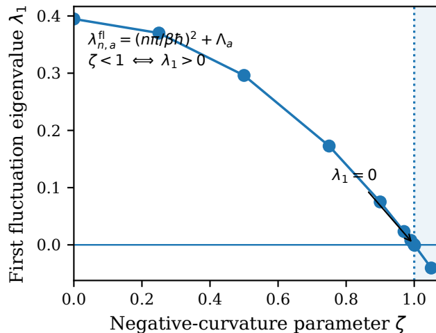
(d) Gaussian existence criterion
