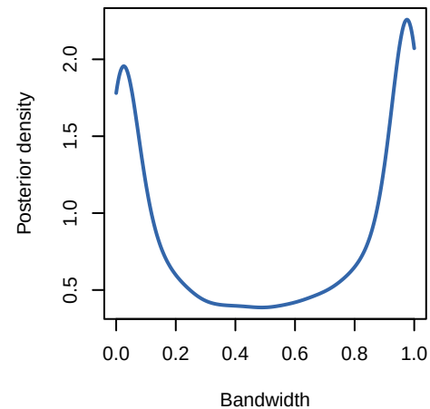
ordinal_2 bandwidth posterior
