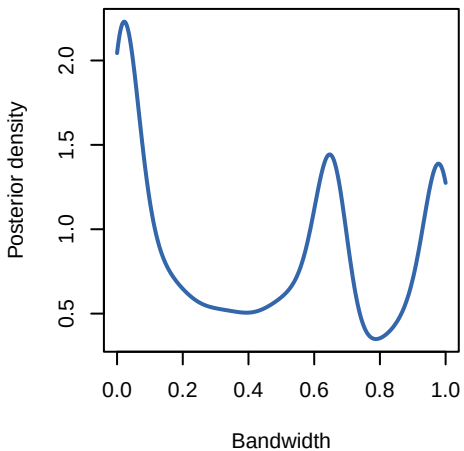
nominal_2 bandwidth posterior
