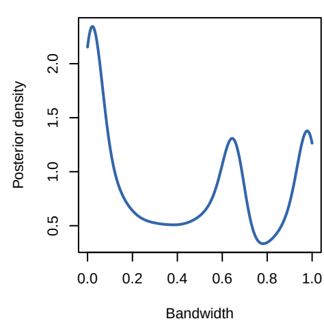
nominal_1 bandwidth posterior
