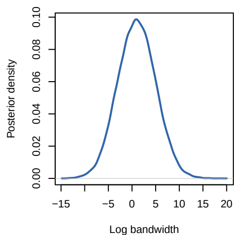
continuous_2 bandwidth posterior
