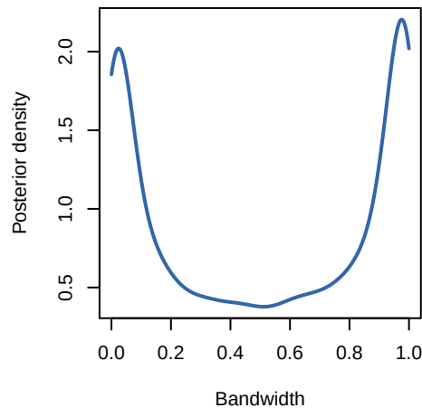
ordinal_1 bandwidth posterior
