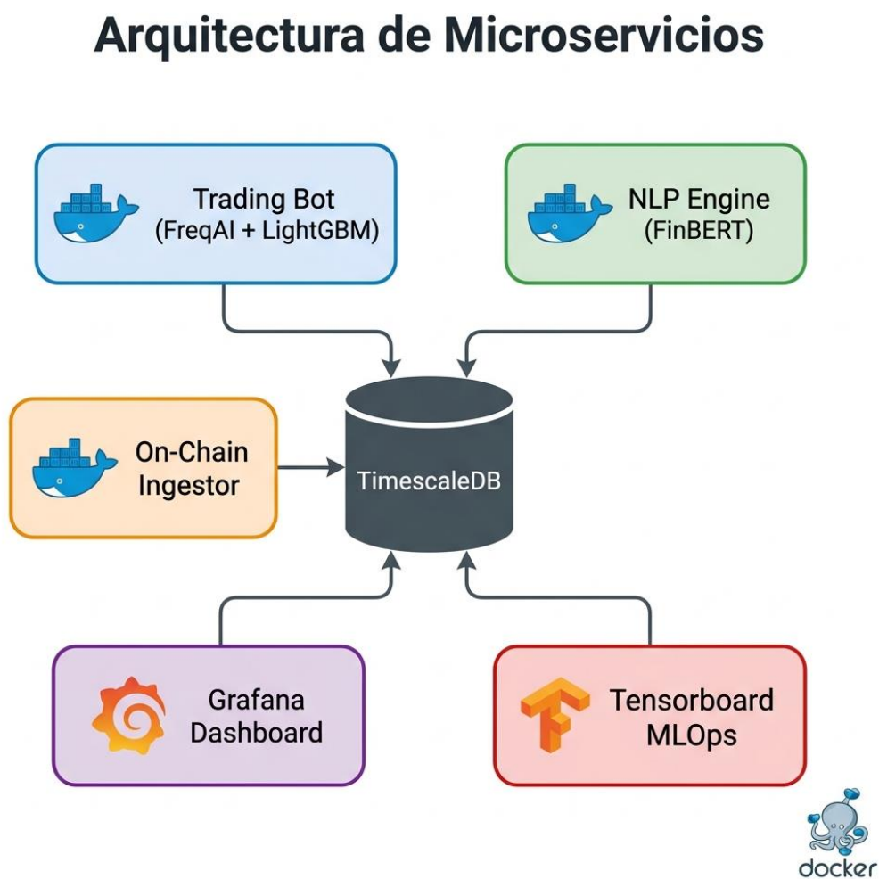
Figura 4.1: Arquitectura de microservicios del sistema
