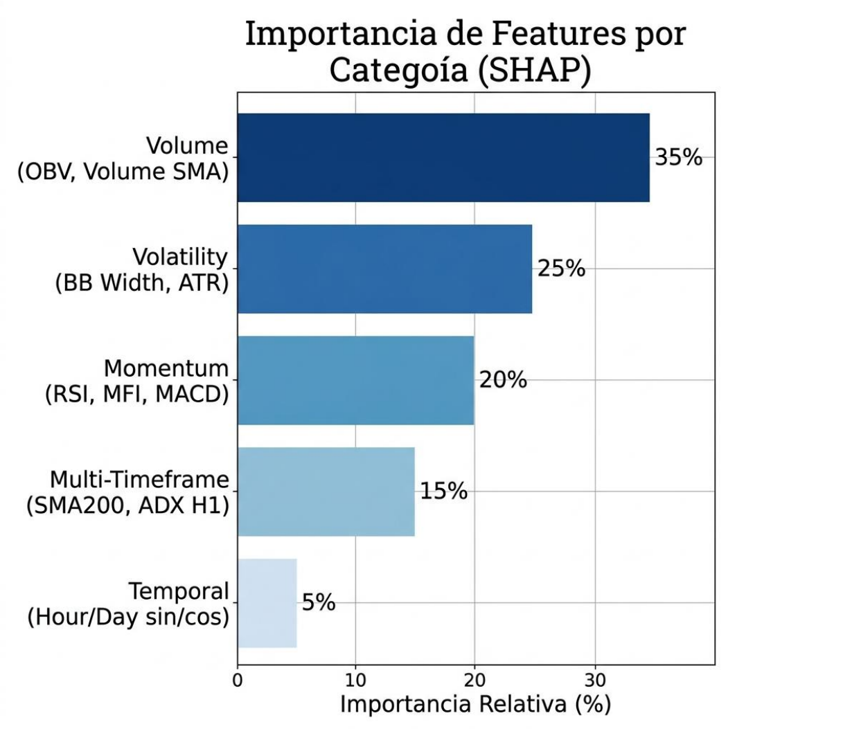
Figura 7.4: Importancia de features por categoría (SHAP)
