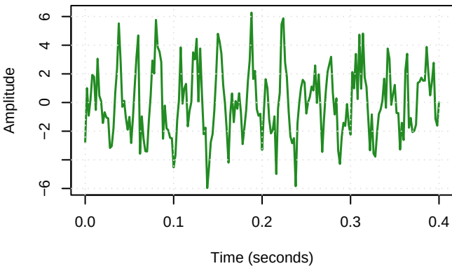
Output EEG Signal y
