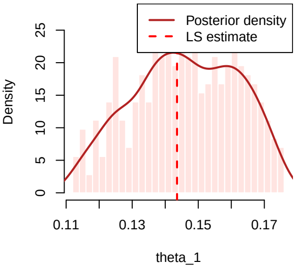
Marginal Posterior – \theta_1
