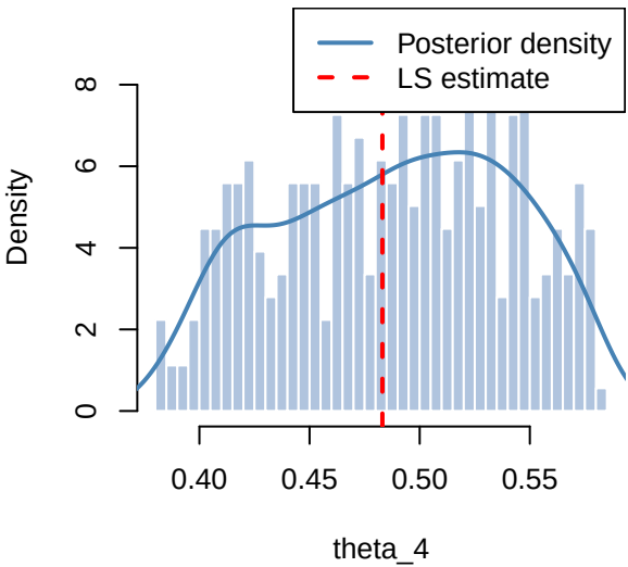
Marginal Posterior – \theta_4
