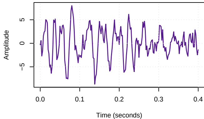
Input EEG Signal x4
