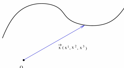
Figura 4.1: Vector Posición.
