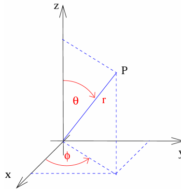
Figura 3.25: Coordenadas Esféricas.
