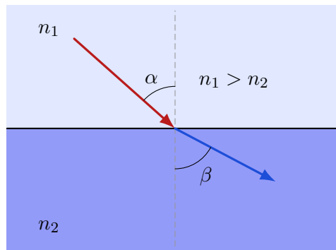
Figura 4: Si n_1 > n_2 , el rayo refractado se aleja de la normal, es decir, \beta > \alpha .
