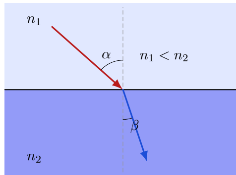
Figura 5: Si n_1 < n_2 , el rayo refractado se acerca a la normal, de modo que \beta < \alpha .
