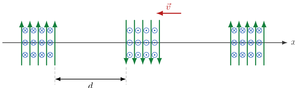
Figura 2: Esquema de la onda en t = 0 . Entre dos regiones consecutivas con campos opuestos hay media longitud de onda.
