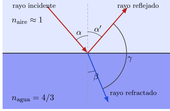
Figura 6: Geometría para un rayo que incide desde el aire hacia el agua.
