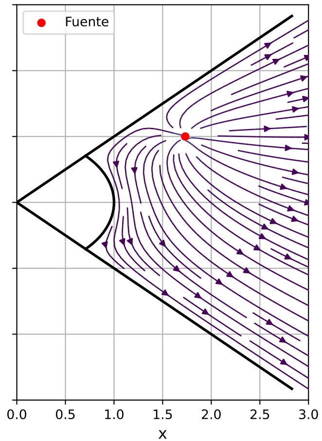
Parte real - i *Parte imaginaria
