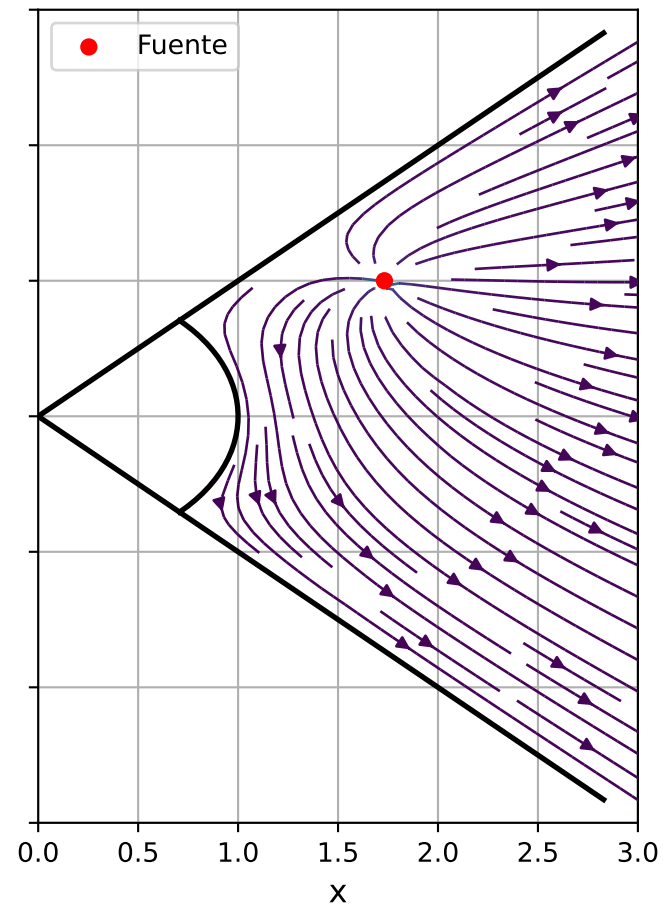
Separación de variables
