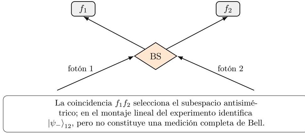
Figura 10. Analizador parcial de Bell mediante divisor de haz. La firma experimental de |\psi_{-}\rangle_{12} es una coincidencia entre los detectores f_1 y f_2 .
