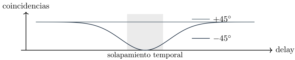
Figura 11. Predicción cualitativa de la Fig. 3 del paper. Para teleportar +45^\circ , el canal ortogonal presenta un dip cerca del retardo nulo, mientras que el canal correcto permanece aproximadamente constante.
