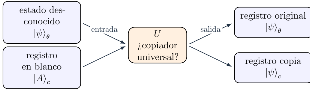
Figura 3. Esquema ideal de una máquina universal de clonado. La imposibilidad aparece al exigir que el mismo operador U funcione para cualquier superposición desconocida.
