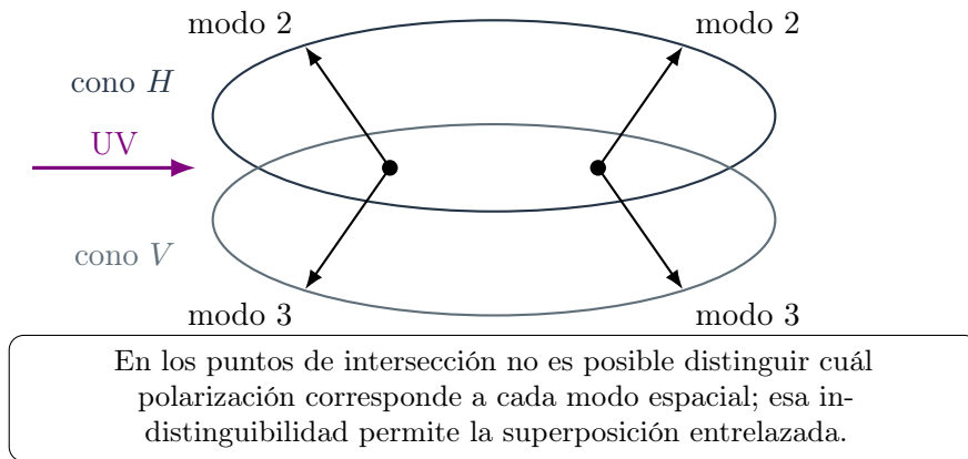
Figura 9. Esquema conceptual de conversión paramétrica descendente tipo II: los puntos de intersección de los conos definen los modos entrelazados.
