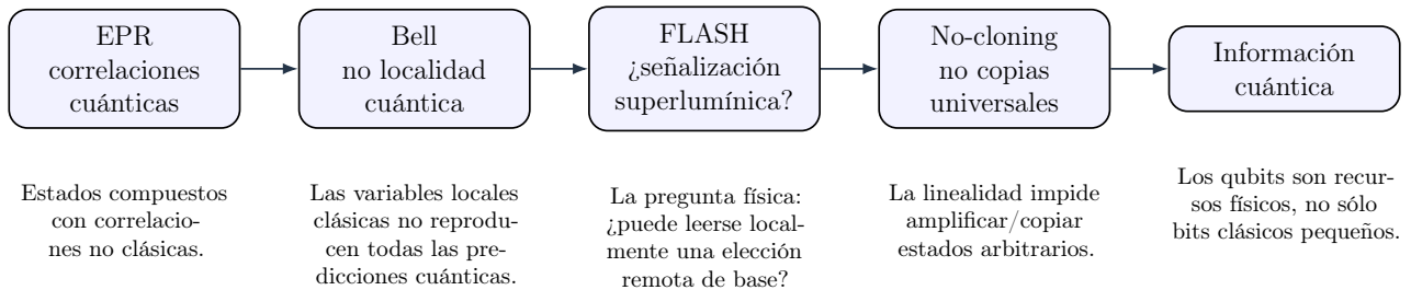
Figura 1. Hilo histórico y conceptual que conecta medición, ensambles, no localidad, no-cloning e información cuántica.
