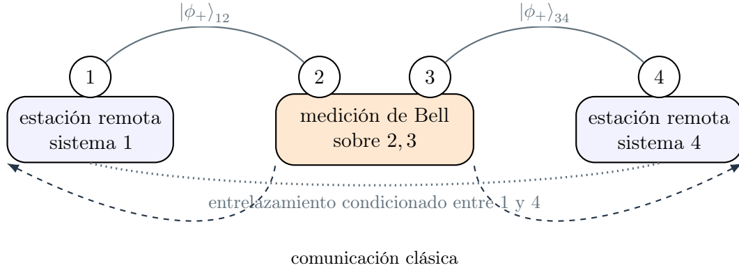
Figura 13. Intercambio de entrelazamiento en la convención 1, 4 para los sistemas remotos y 2, 3 para los sistemas medidos. La correlación remota queda condicionada al resultado de la medición central.
