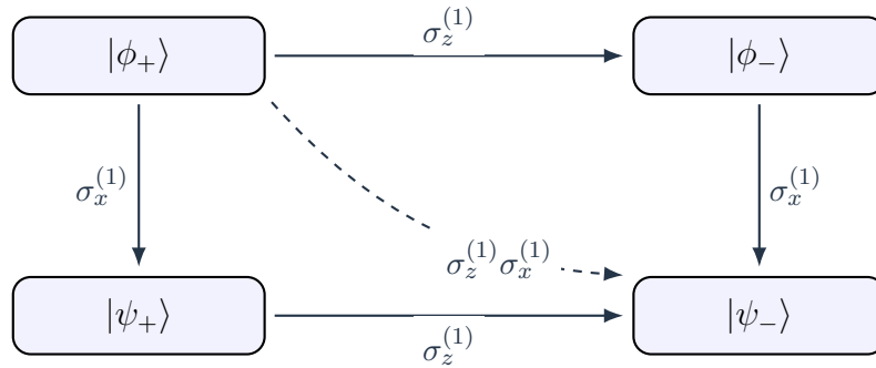
Figura 6. Los cuatro estados de Bell se obtienen unos de otros mediante operaciones locales de Pauli sobre uno de los qubits.
