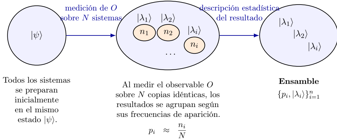
Figura 2. Esquema del paso desde un estado inicial puro hacia un ensamble estadístico de autoestados luego de medir el observable O . La figura fue reubicada directamente en el sistema de coordenadas de TikZ, de modo que el conjunto completo queda centrado respecto del texto.
