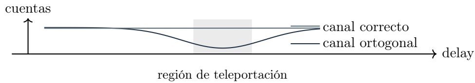
Figura 12. Redibujo cualitativo de las Figs. 4 y 5 del paper. El canal ortogonal presenta un dip en la región de solapamiento, mientras que el canal compatible con la polarización teleportada permanece alto.
