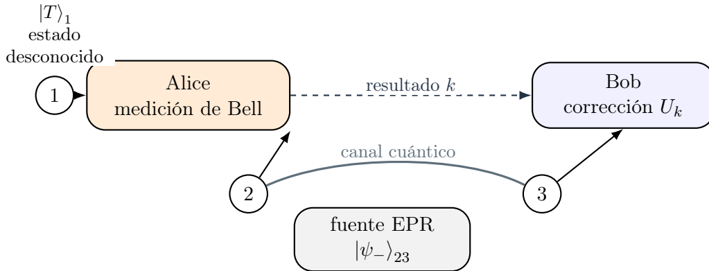
Figura 7. Esquema conceptual de teleportación cuántica. El par EPR constituye el canal cuántico; el resultado de la medición de Bell se transmite por un canal clásico.
