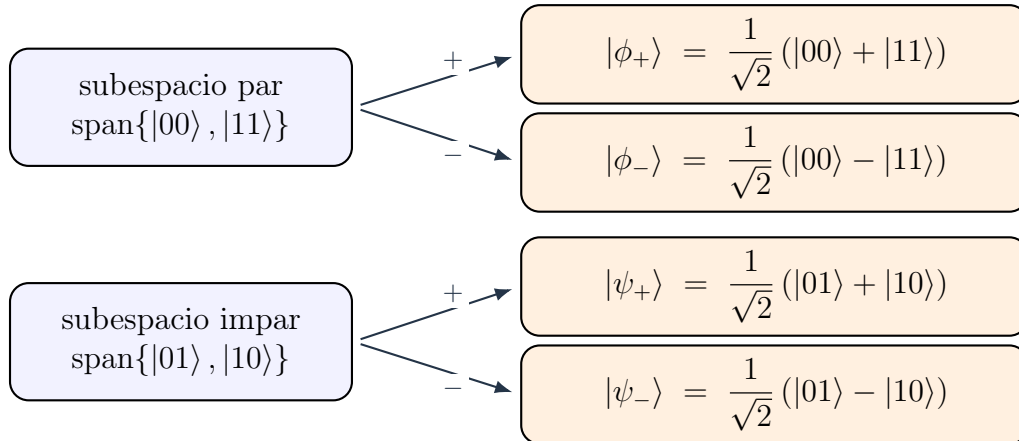
Figura 4. La base de Bell se obtiene combinando los subespacios de paridad par e impar con signos relativos. Esta organización evita identificar los estados entrelazados con estados producto individuales.
