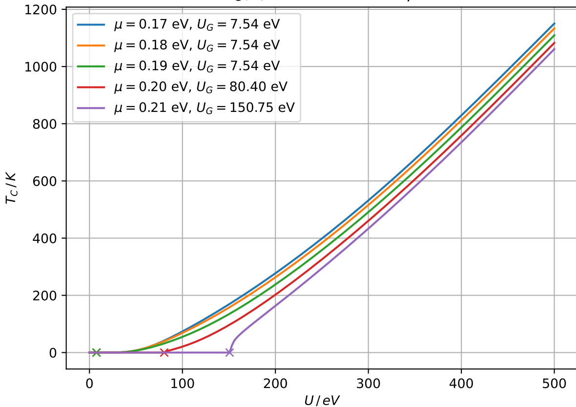
T_C(U) für verschiedene \mu
