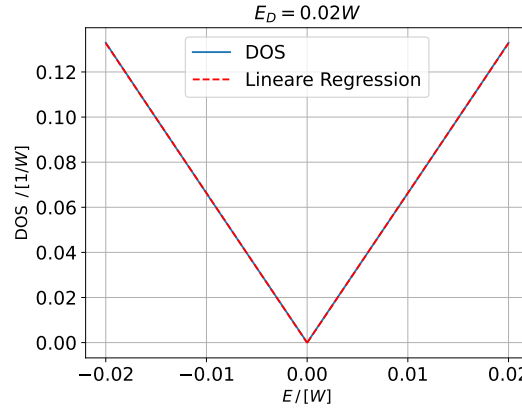
Abbildung 4.3: Vergleich der DOS des Bienenwabengitters mit einer linearen Regression im Bereich [-E_D, E_D] für E_D = 0,02 W . Die lineare Regression liefert A \approx 6,6447 W^{-2} .
