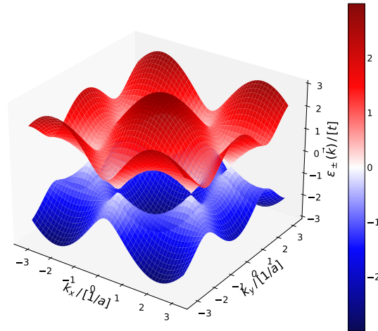
Abbildung 2.2: Plot der TB-Bandstruktur des Bienenwabengitters (3.33). Dieser Plot wurde mit matplotlib [7] erstellt.
