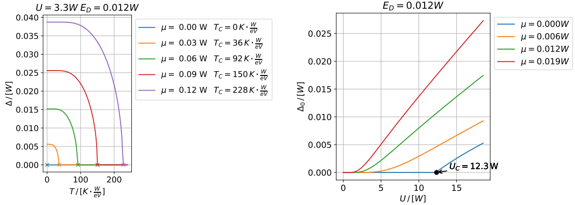
Abbildung 4.2: Abhängigkeiten des Ordnungsparameters \Delta für verschiedene Dotierungsstärken \mu in Einheiten der Bandbreite W . Links in Abhängigkeit von der Temperatur T bei festen Parametern U = 3,3 W und E_D = 12 \cdot 10^{-3} W und rechts für verschiedene Kopplungsstärken U bei T = 0 und E_D = 12 \cdot 10^{-3} W . Der Ordnungsparameter verschwindet oberhalb einer kritischen Temperatur T_C , die stark von \mu abhängig ist und geht bei endlichem \mu für kleine U exponentiell fallend gegen null. Für \mu = 0 bildet sich ein endliches \Delta_0 erst oberhalb der kritischen Kopplung U_C = 12,3 W aus.
