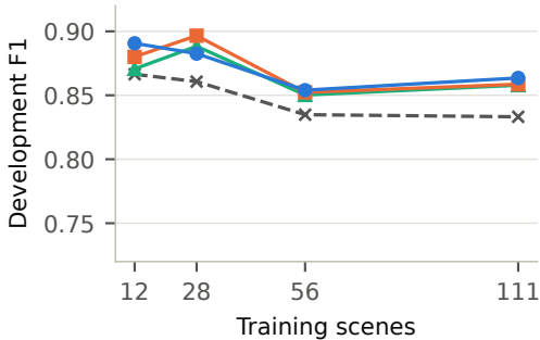
ViT-B/16
