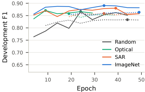
ViT-B/16
