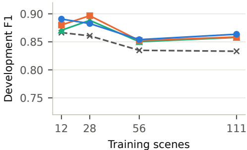
ViT-B/16
