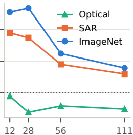
ConvNeXt-V2-B
