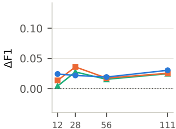
ViT-B/16
