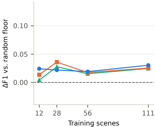
ViT-B/16
