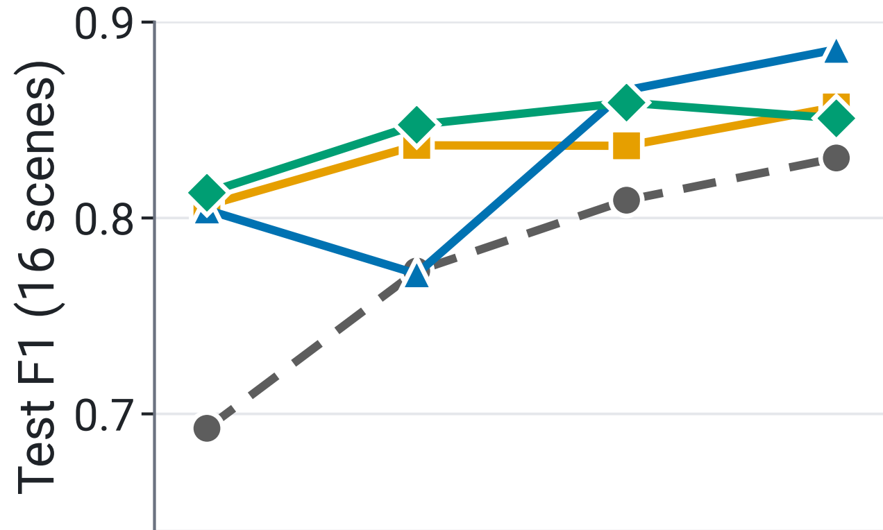
ViT-B/16
