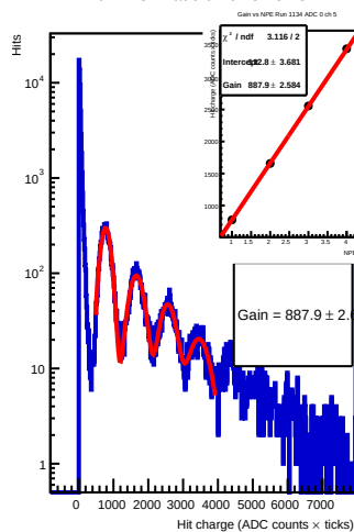
Run 1134 - adc 0 - ch 5 - 57.5V
