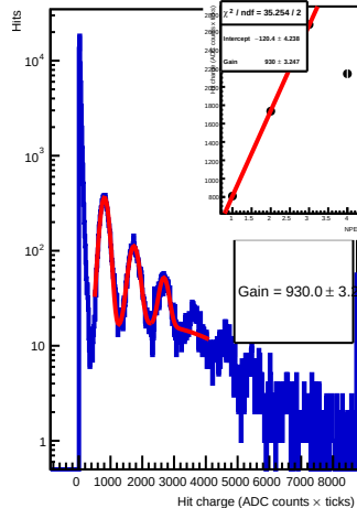
Run 1135 - adc 0 - ch 4 - 58.0V
