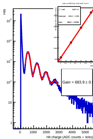
Run 1131 - adc 0 - ch 5 - 56.0V
