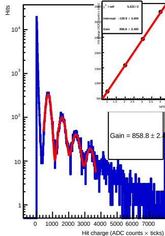
Run 1134 - adc 0 - ch 6 - 57.5V
