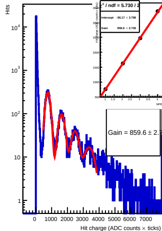
Run 1134 - adc 0 - ch 4 - 57.5V
