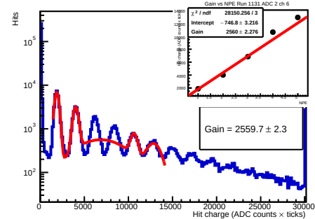
Run 1131 - adc 2 - ch 6 - 56.0V
