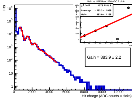
Run 1126 - adc 2 - ch 6 - 53.5V
