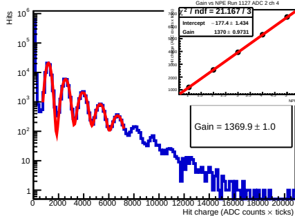
Run 1127 - adc 2 - ch 4 - 54.5V
