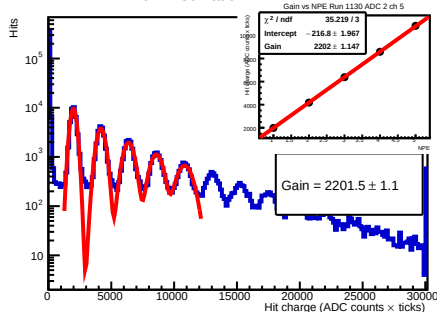
Run 1130 - adc 2 - ch 5 - 55.5V
