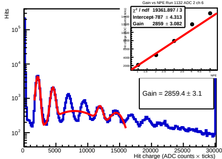
Run 1132 - adc 2 - ch 6 - 56.5V
