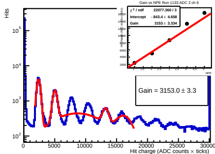
Run 1133 - adc 2 - ch 6 - 57.0V
