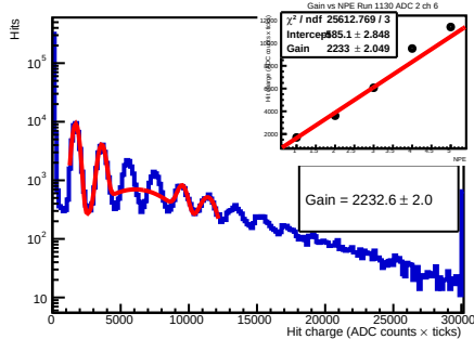
Run 1130 - adc 2 - ch 6 - 55.5V
