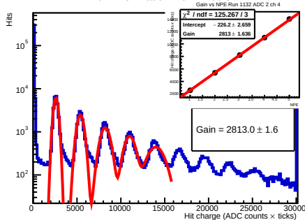
Run 1132 - adc 2 - ch 4 - 56.5V
