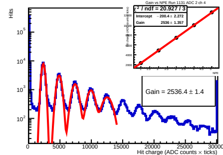
Run 1131 - adc 2 - ch 4 - 56.0V
