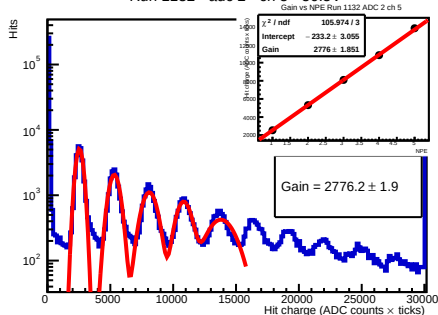
Run 1132 - adc 2 - ch 5 - 56.5V
