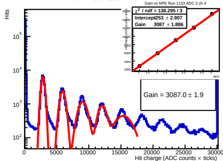
Run 1133 - adc 2 - ch 4 - 57.0V
