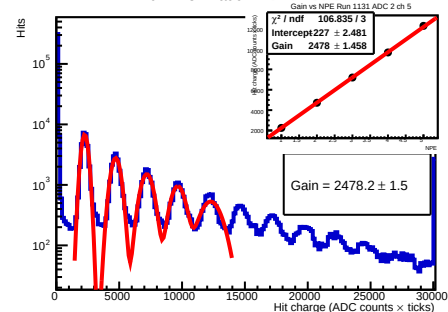
Run 1131 - adc 2 - ch 5 - 56.0V
