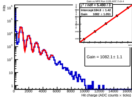
Run 1126 - adc 2 - ch 4 - 53.5V
