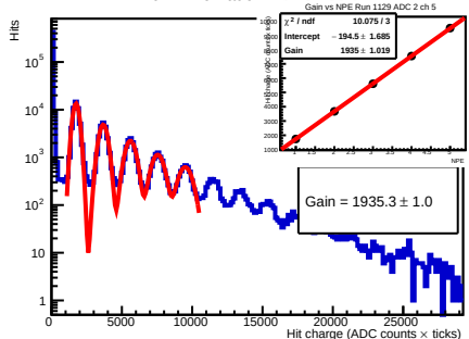
Run 1129 - adc 2 - ch 5 - 55.0V
