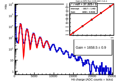
Run 1128 - adc 2 - ch 4 - 54.5V
