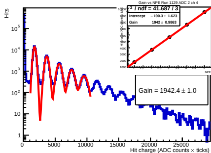
Run 1129 - adc 2 - ch 4 - 55.0V
