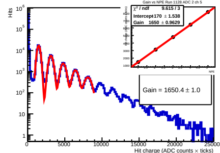
Run 1128 - adc 2 - ch 5 - 54.5V
