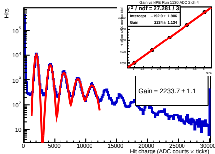
Run 1130 - adc 2 - ch 4 - 55.5V
