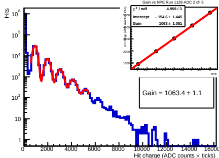
Run 1126 - adc 2 - ch 5 - 53.5V
