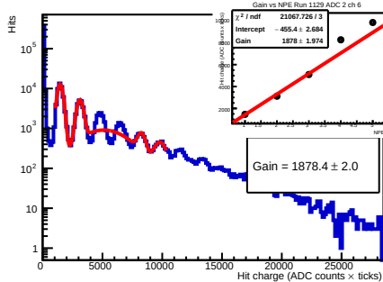
Run 1129 - adc 2 - ch 6 - 55.0V
