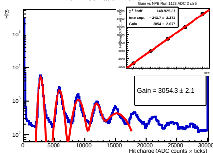
Run 1133 - adc 2 - ch 5 - 57.0V
