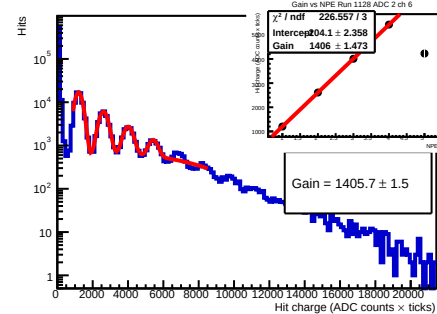
Run 1128 - adc 2 - ch 6 - 54.5V
