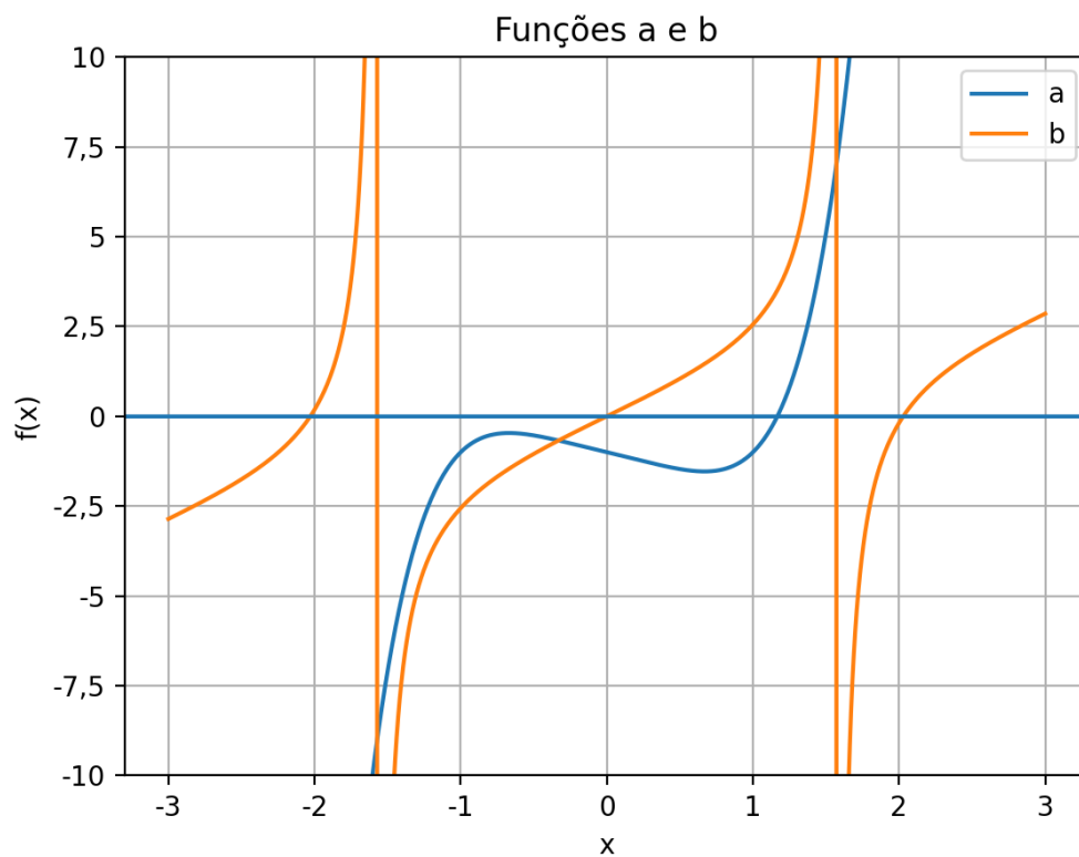
Figura 7: Comportamento das funções dos itens (a) e (b).
