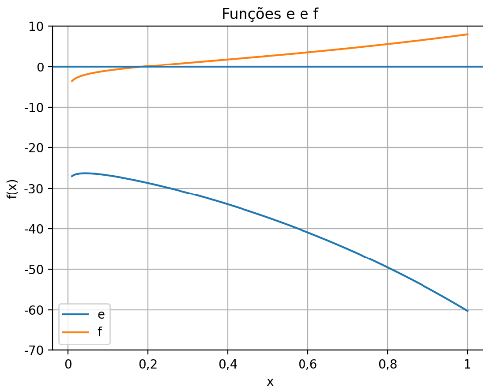
Figura 9: Comportamento das funções dos itens (e) e (f).
