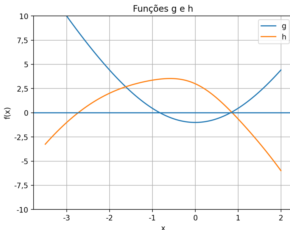
Figura 10: Comportamento das funções dos itens (g) e (h).
