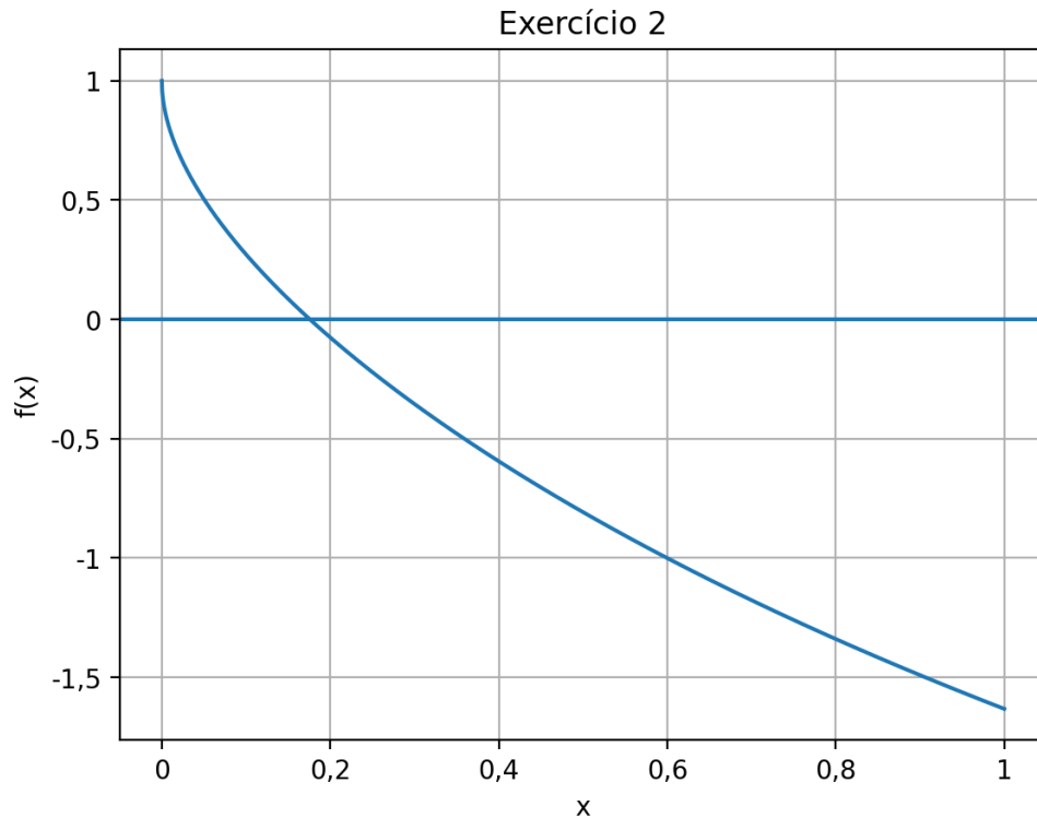
Figura 11: Comportamento da função f(x) = e^{-x} - 2\sqrt{x} no intervalo [0, 1] .
