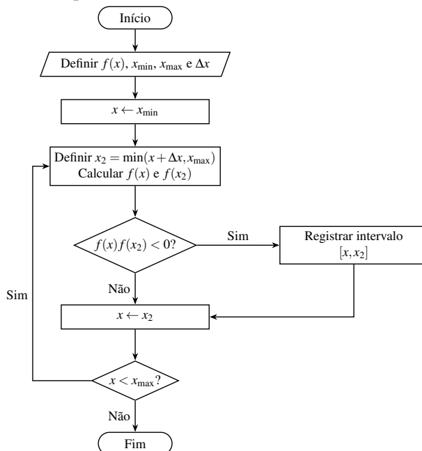
Figura 1: Fluxograma da busca incremental.
