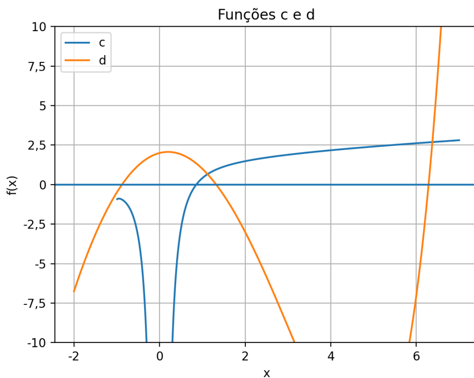
Figura 8: Comportamento das funções dos itens (c) e (d).
