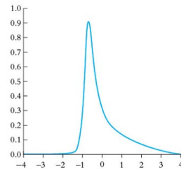
(d) Skewness = 0.6, kurtosis = 5
