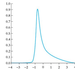
(d) Skewness = 0.6, kurtosis = 5
