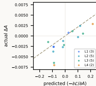
(d) Raw gradient r = 0.796
