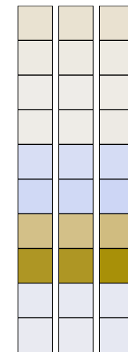
\hat{\theta}^{\Lambda^{(t)}}
