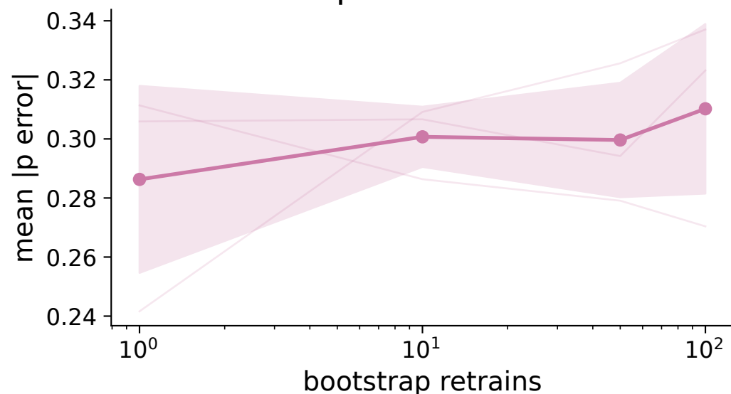
Exponent Error
