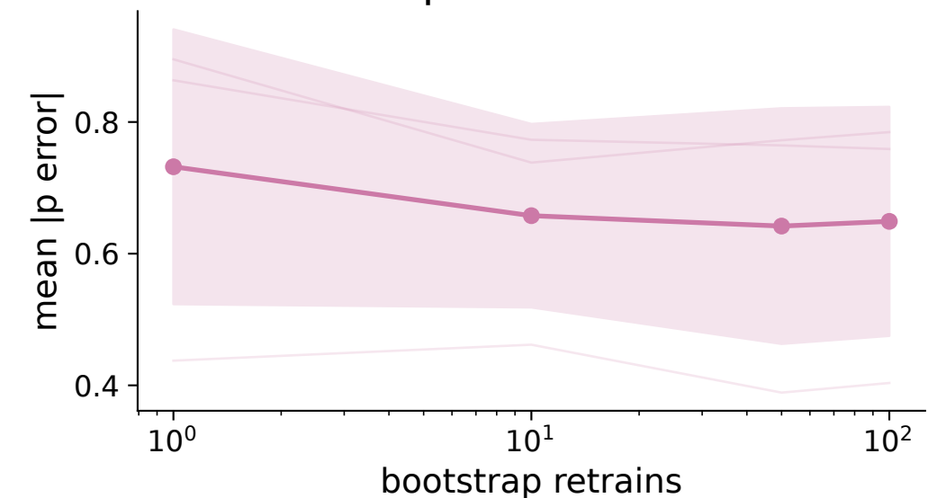
Exponent Error
