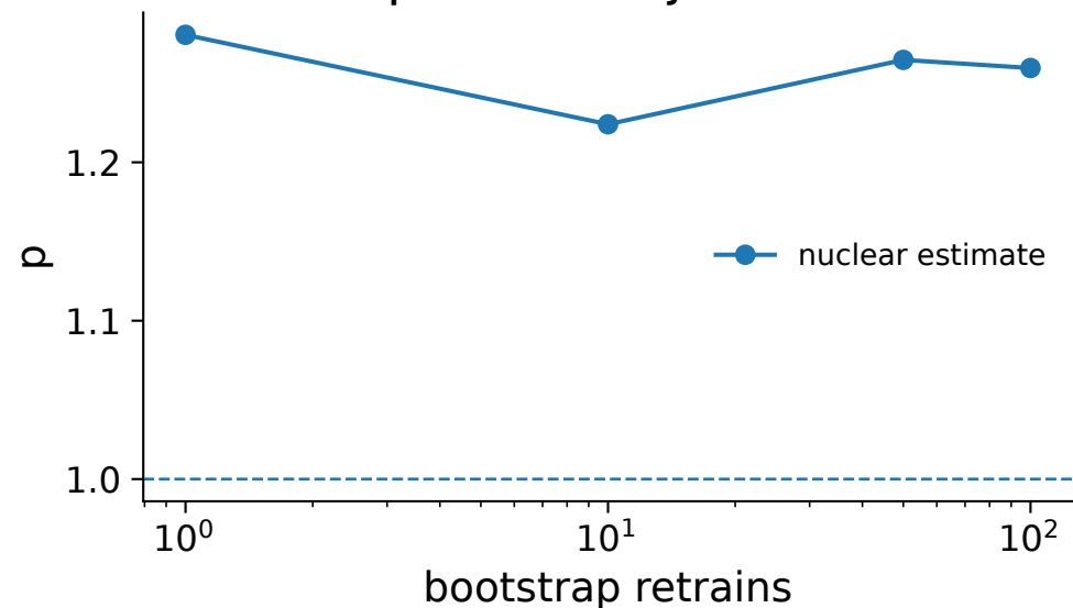
Exponent Trajectories
