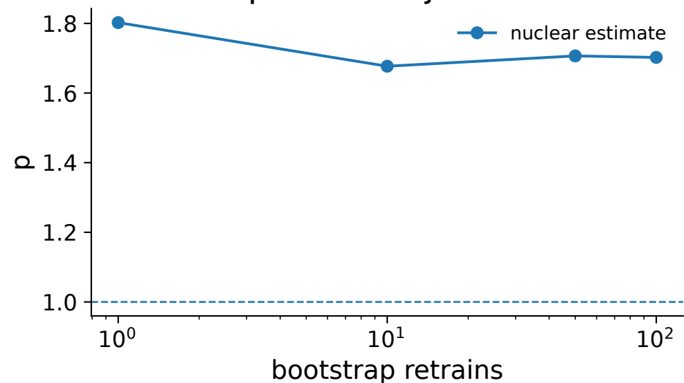
Exponent Trajectories
