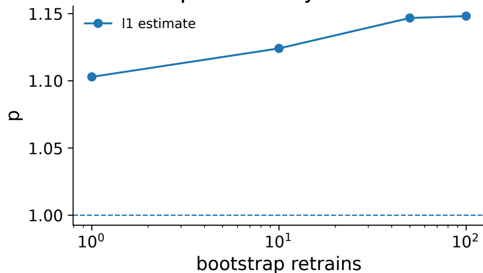
Exponent Trajectories
