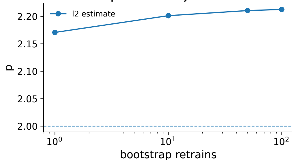
Exponent Trajectories
