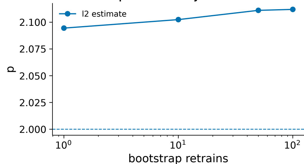
Exponent Trajectories
