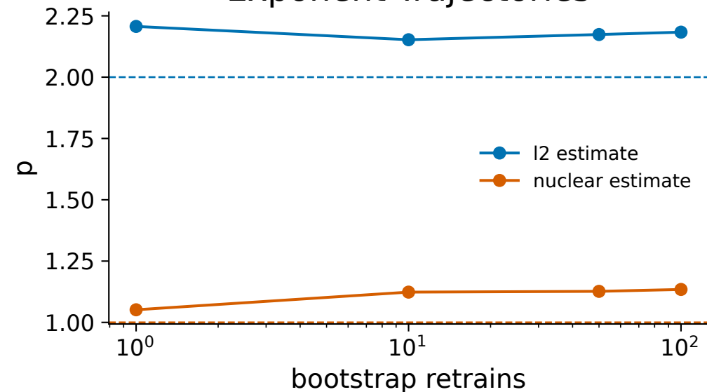
Exponent Trajectories
