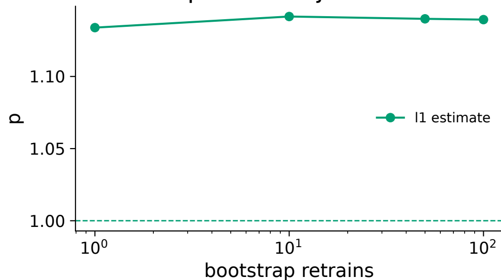
Exponent Trajectories
