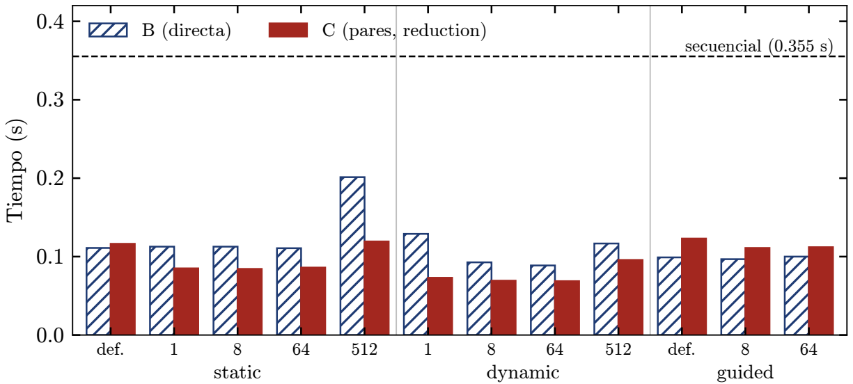
Figura 2: Tiempo con 8 hilos según el schedule y el chunk . La línea discontinua indica el tiempo de la versión secuencial.
