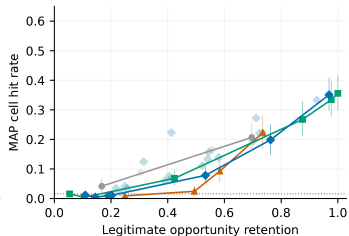
Geolife
