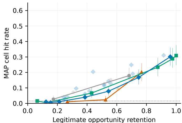
Geolife
