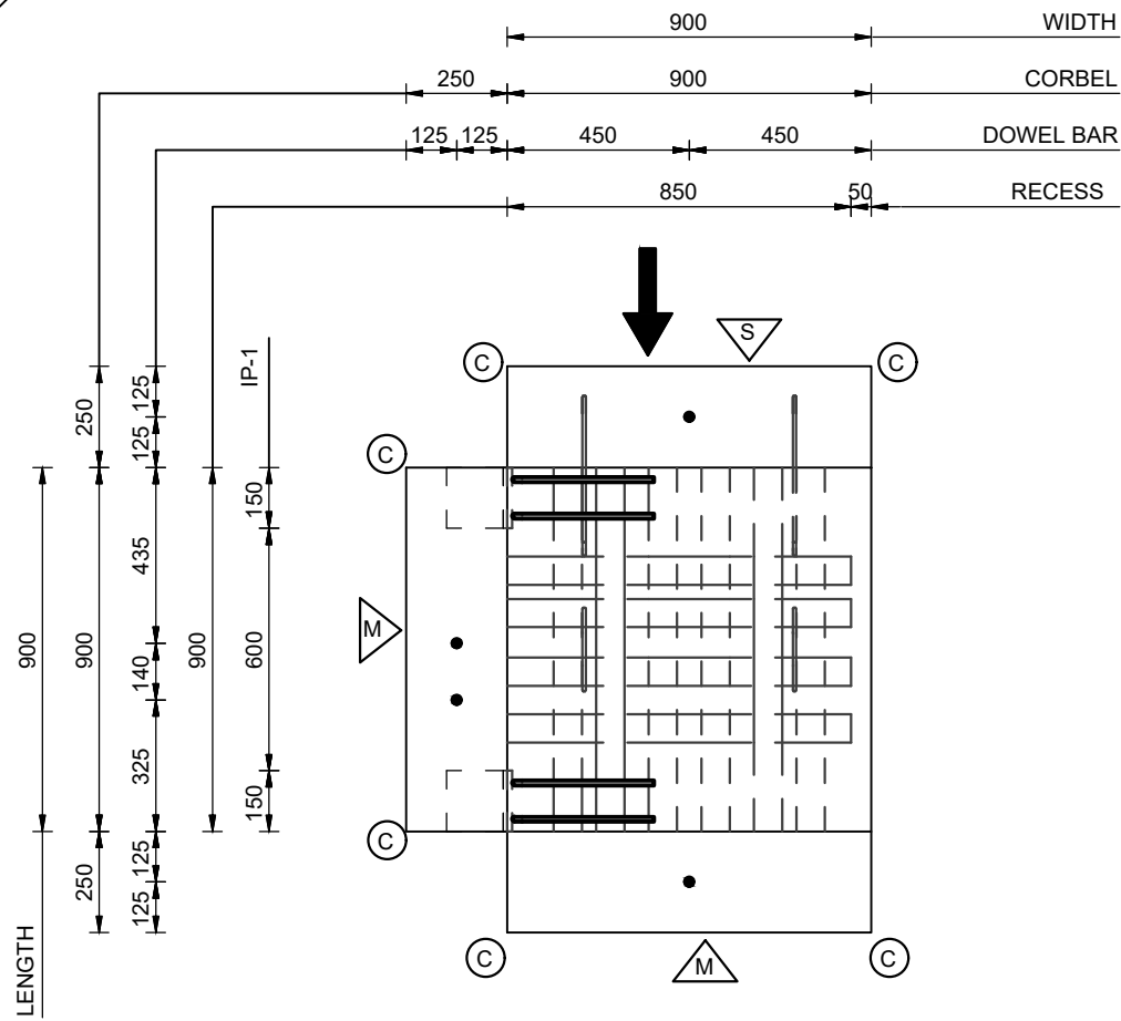
SECTION B SCALE - 1 : 20
