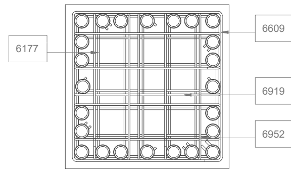
SECTION SCALE - 1 : 20
