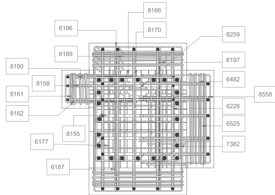
SECTION SCALE - 1 : 20
