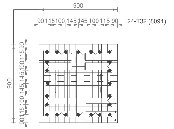
SECTION SCALE - 1 : 25
