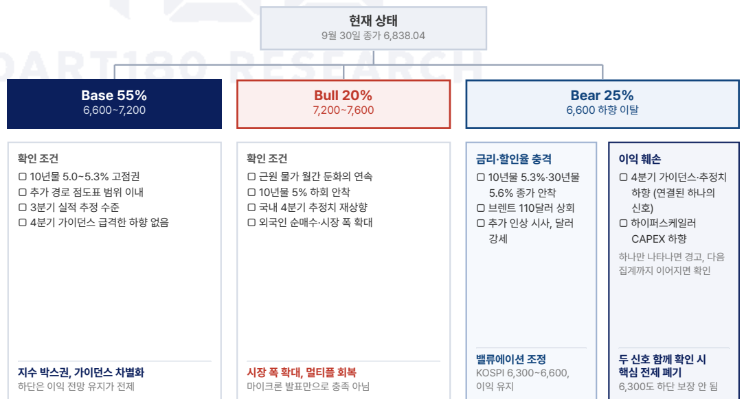
그림 7. Scenario Tree
