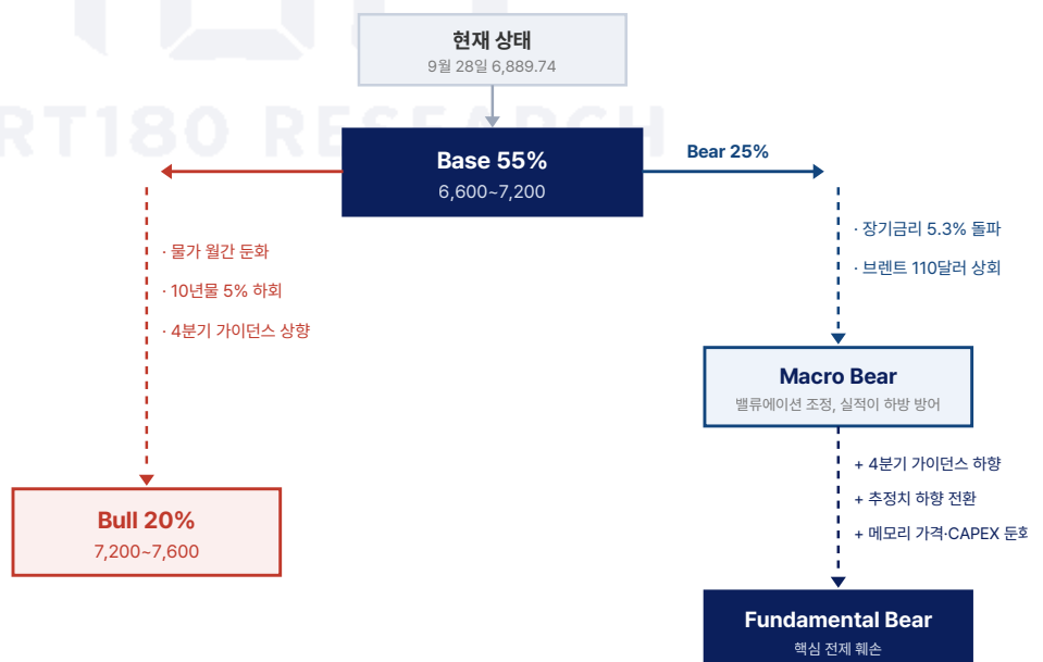
그림 6. Scenario Tree
