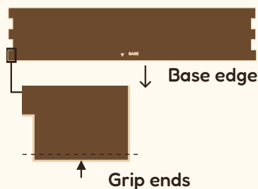
3 fingers per end
