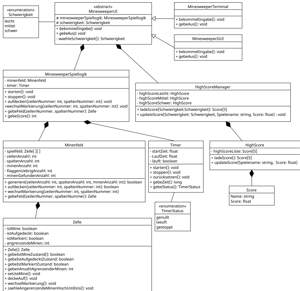
Abbildung 1: Das Klassendiagramm für Minesweeper
