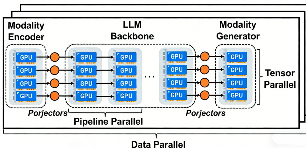
图 1.3 使用 Megatron-LM 框架训练多模态大语言模型
