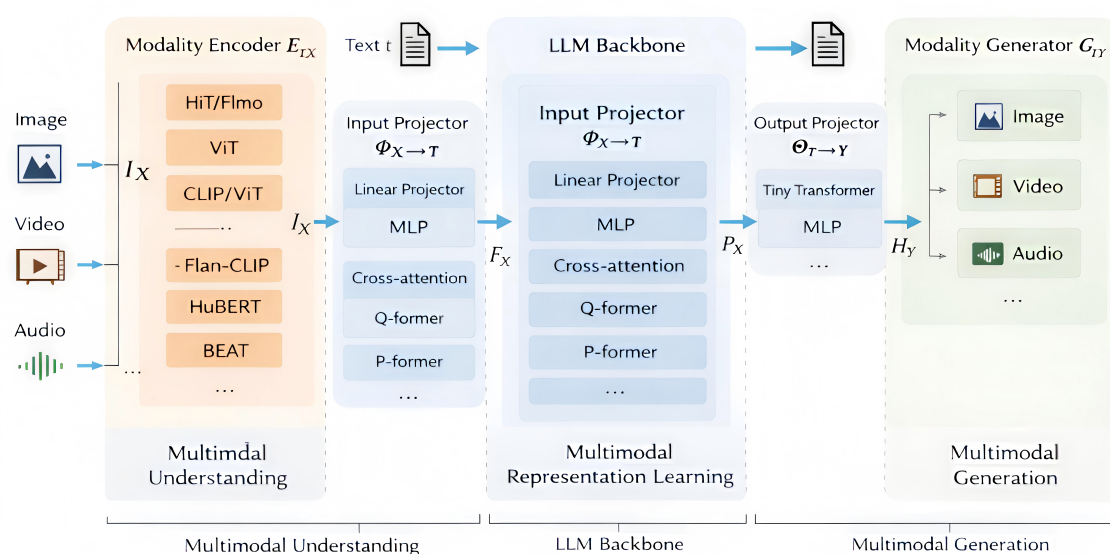
图 1.1 多模态大语言模型的核心组成部分
