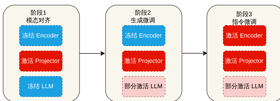
图 2.1 MLLM 多阶段训练中典型模块冻结
