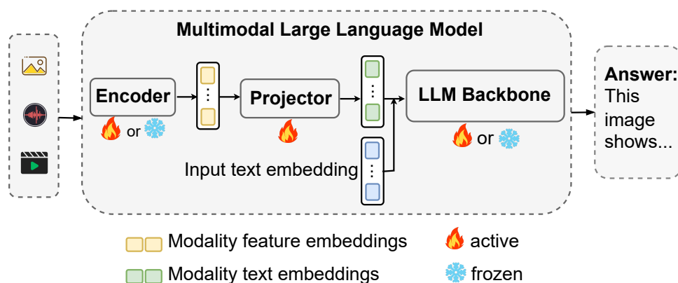
图 3.1 主流 MLLMs 的编码器—投影层—LLM 结构及冻结方式。
