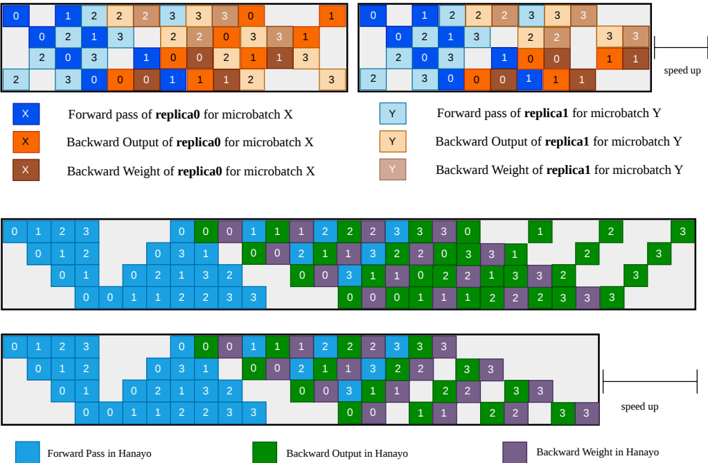
图 3.7 提前终止在其它流水线调度机制上的适用性。上：Chimera（双向流水线）；下：Hanayo（波式流水线）。
