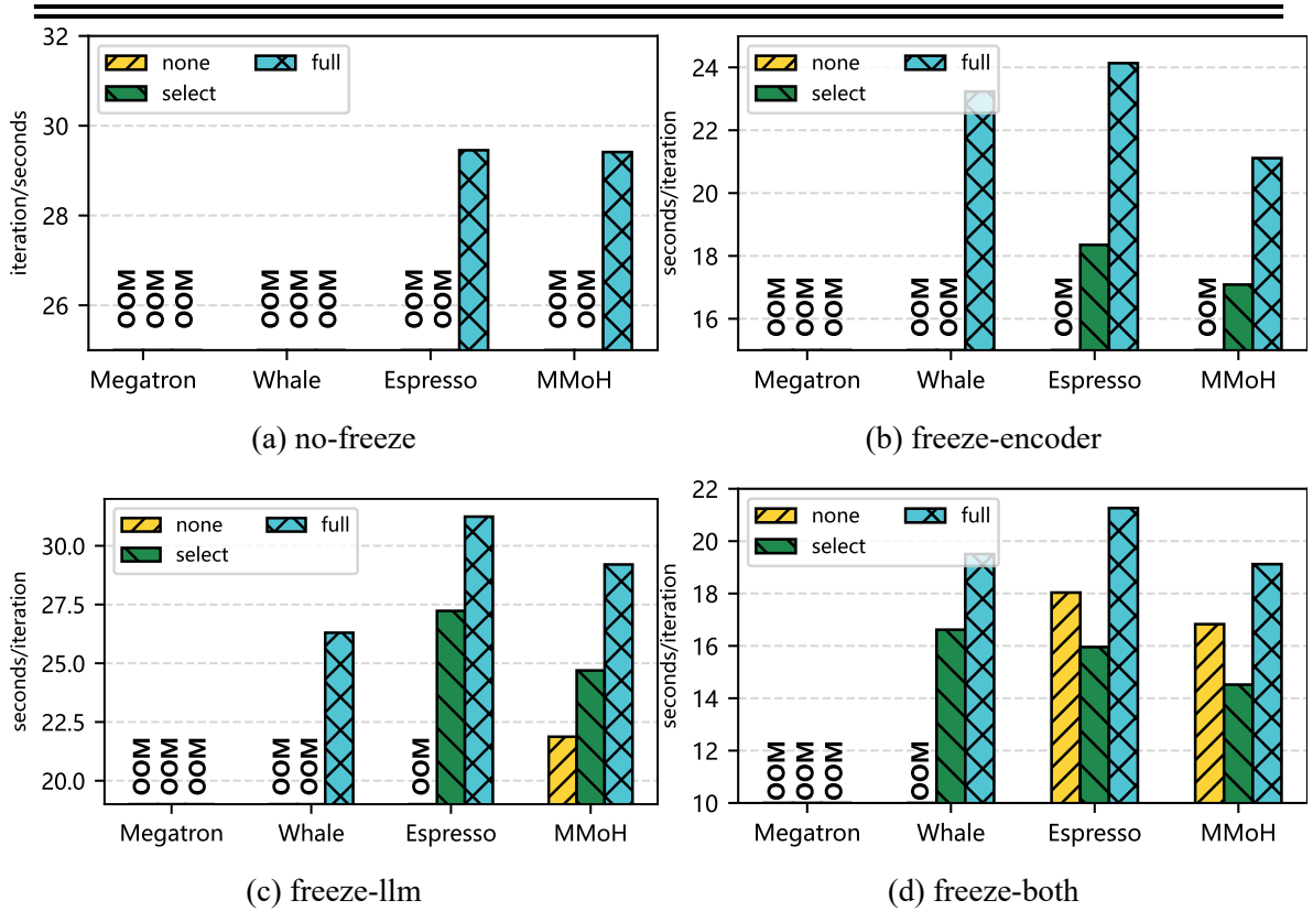
图 4.4 不同冻结策略下各框架迭代时间对比（自左至右、自上至下依次为 no-freeze、freeze-encoder、freeze-llm、freeze-both）。
