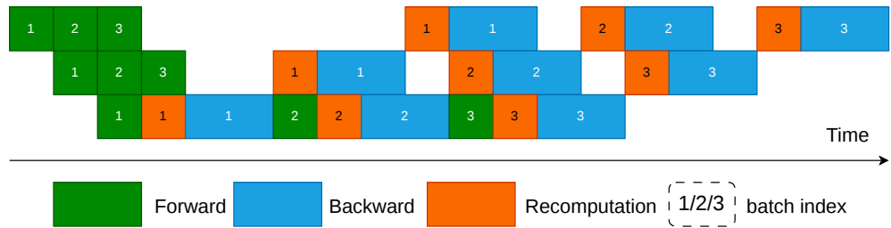
图 2.7 重计算示意图
