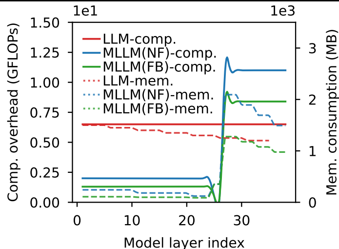
图 3.2 LLM 与 MLLM-3B 各层计算开销与显存占用的变化趋势
