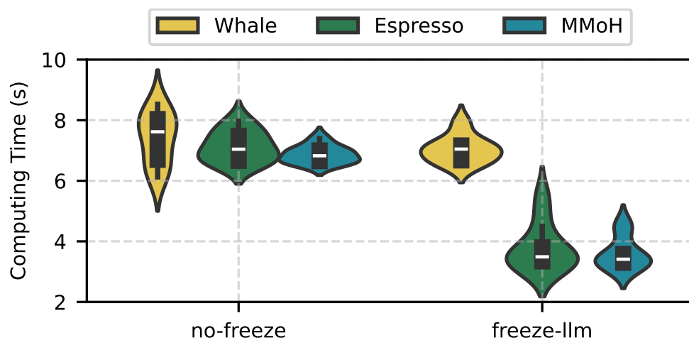
图 3.9 MMoH 与 Whale、Espresso 在 MLLM-12B 上的负载均衡对比
