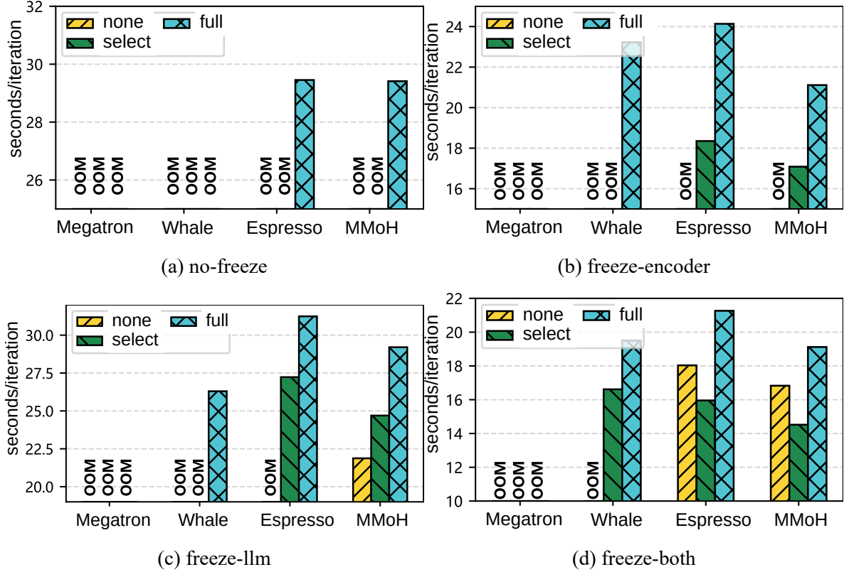
图 4.4 不同冻结策略下各框架迭代时间对比
