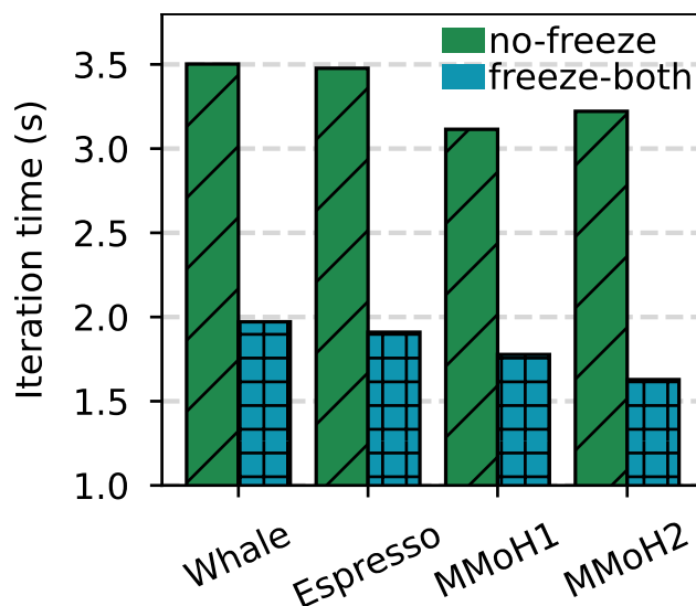
图 3.3 不同并行策略在两种冻结场景下训练 MLLM-3B 的迭代时间
