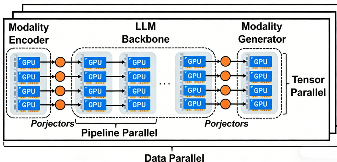
图 1.3 Megatron-LM 训练多模态大语言模型的典型并行配置
