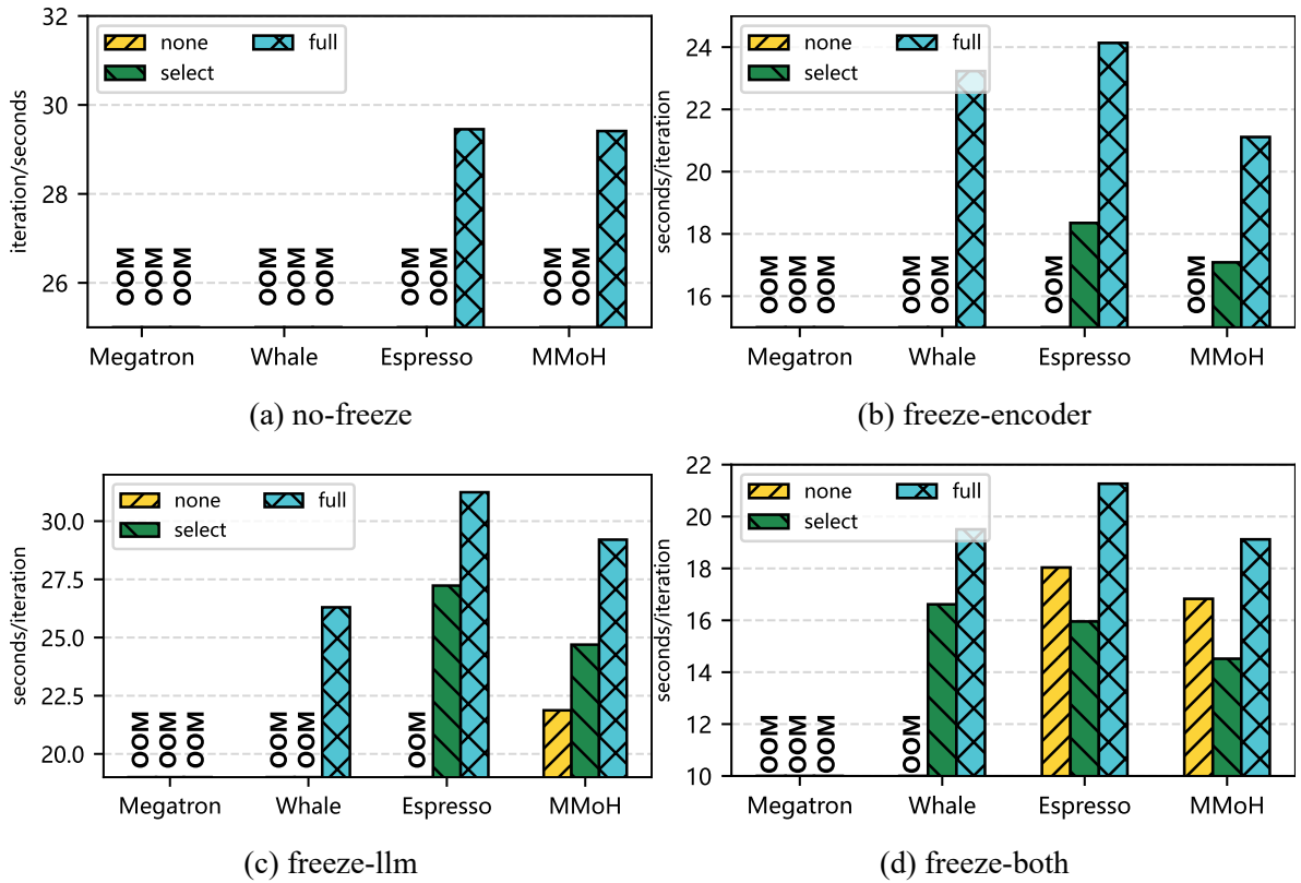
图 4.4 不同冻结策略下各框架迭代时间 (seconds/iteration) 对比 (自左至右、自上至下依次为 no-freeze、freeze-encoder、freeze-llm、freeze-both)。
