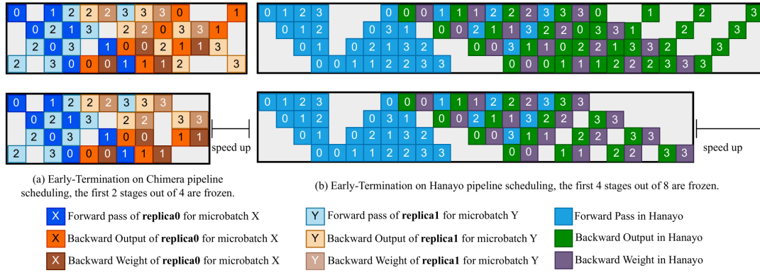
图 3.7 提前终止在其它流水线调度机制上的适用性。左：Chimera；右：Hanayo。前向时间假设各流水级一致，反向时间差异来自冻结流水级；提前终止可同样应用于连续冻结前缀。
