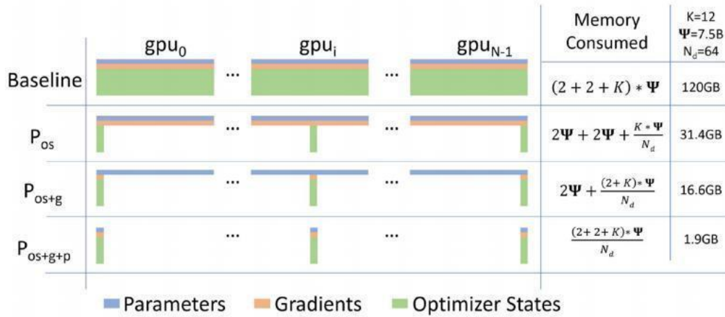
图 2.6 零冗余优化器 ZeRO 示意
